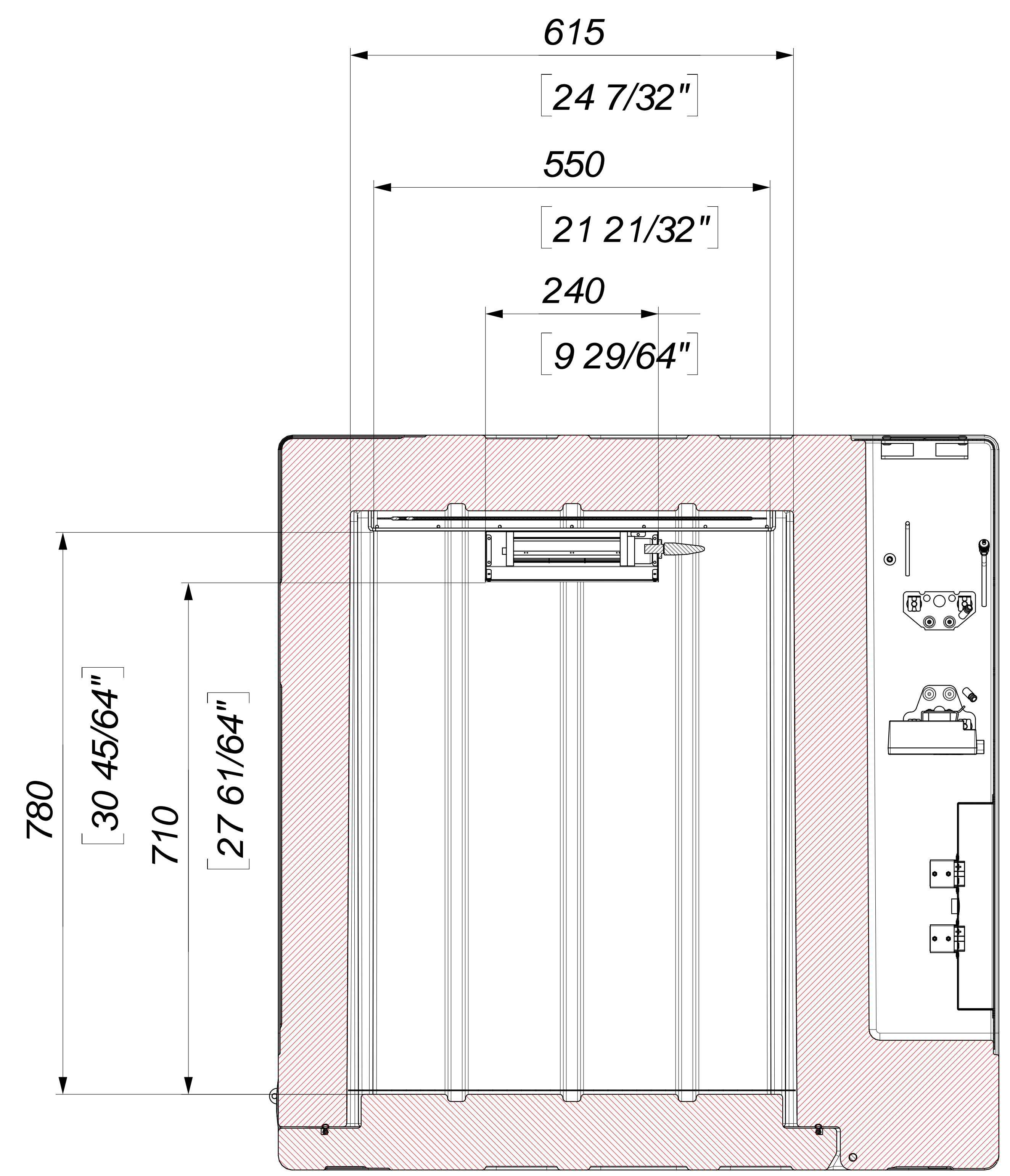
Sezione F-F SCALE 1 : 4
