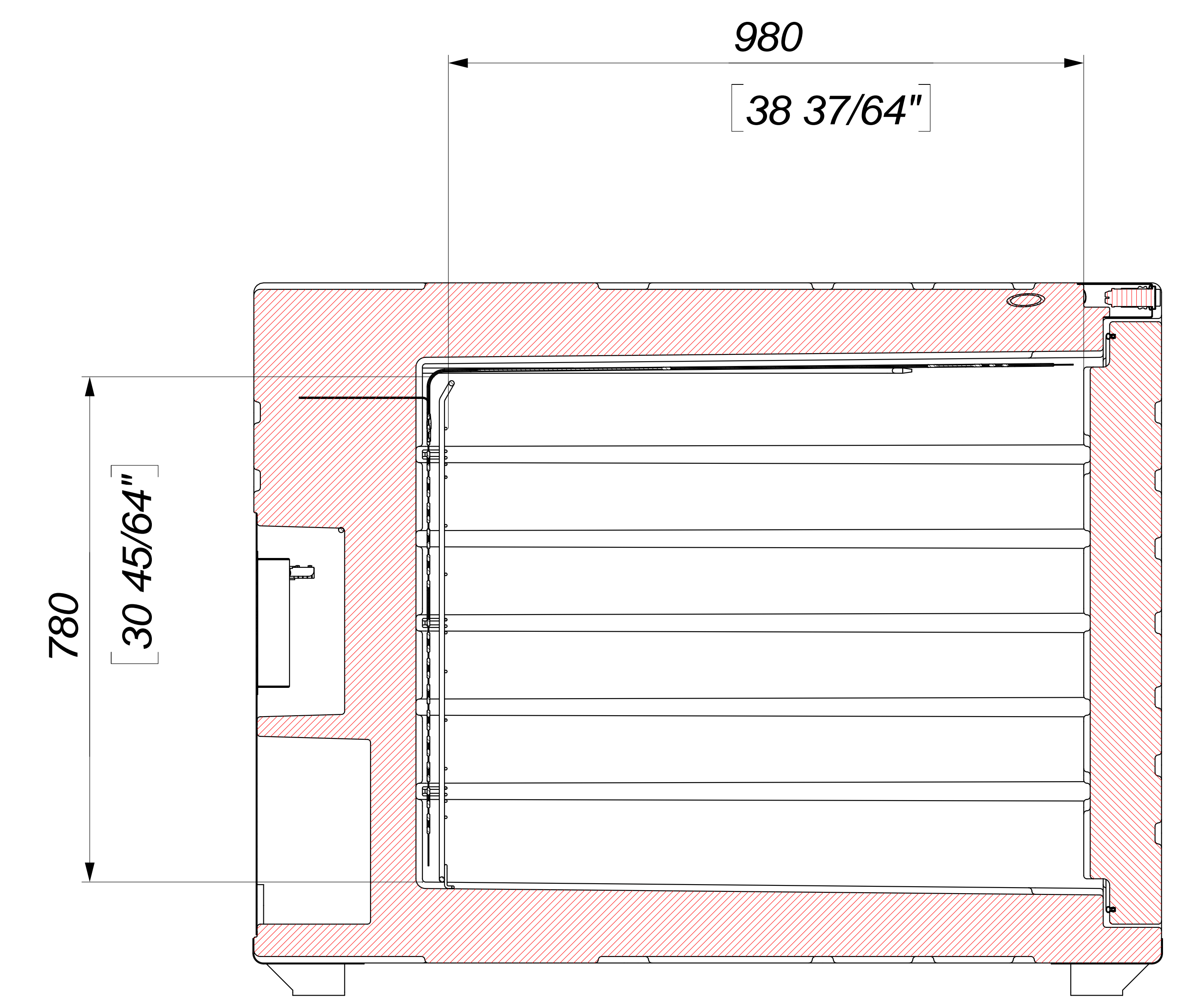
Sezione E-E SCALE 1:5
