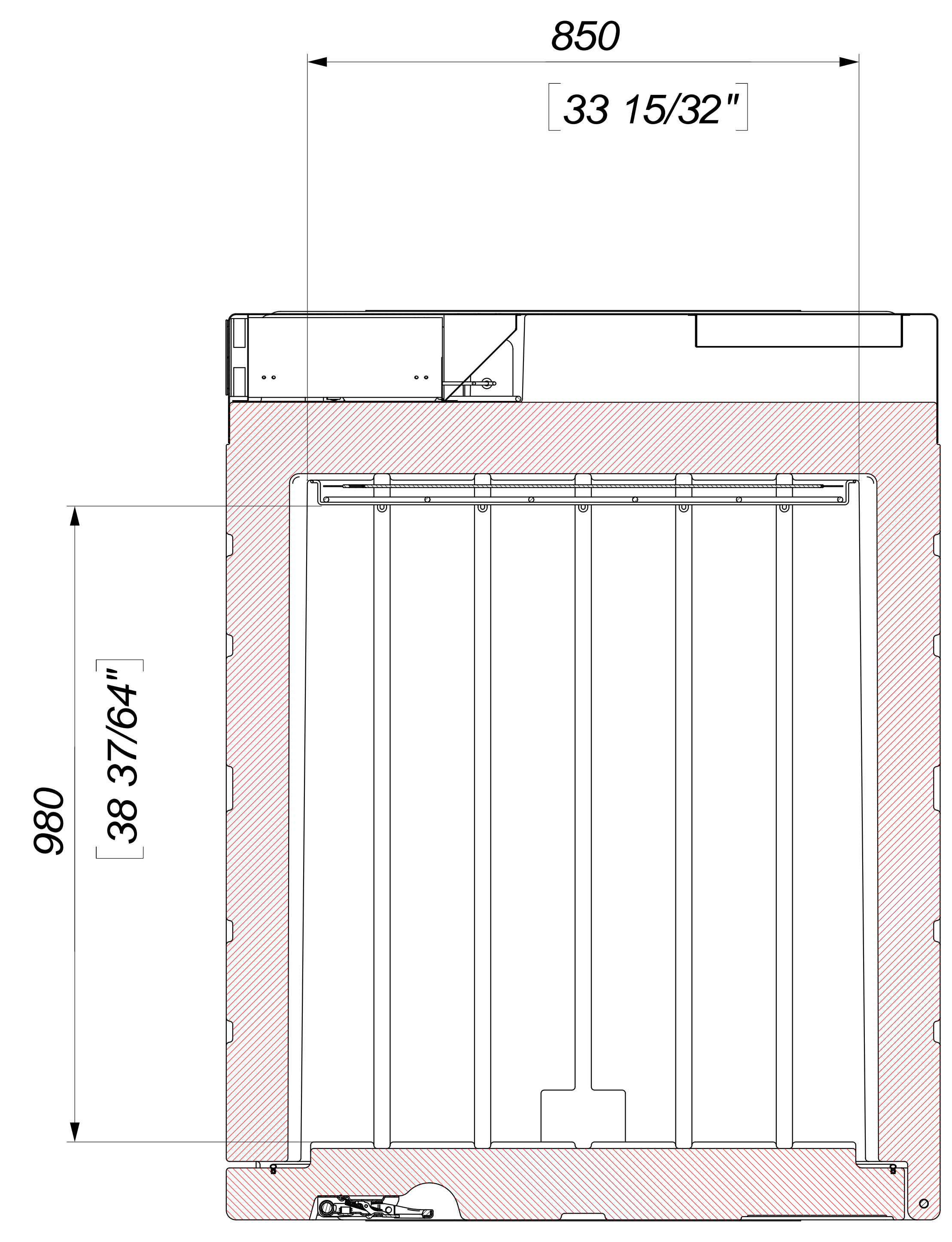
Sezione F-F SCALE 1:5
